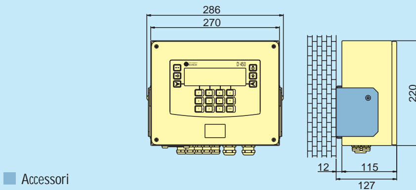
D 450 versione da parete
