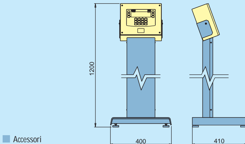
D 450 versione con piedistallo
