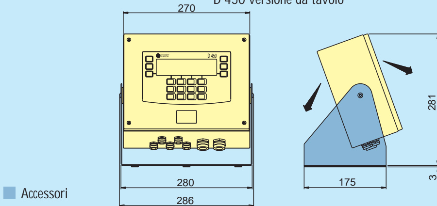
D 450 versione da tavolo
