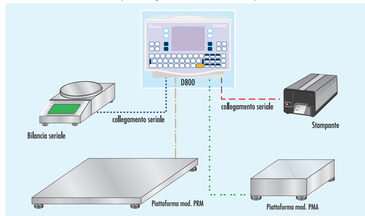
Esempio di configurazione a tre bilance con stampante
